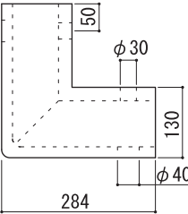
CDL-1315(出隅コーナー)
