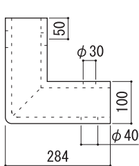
CDL-1010(出隅コーナー)
